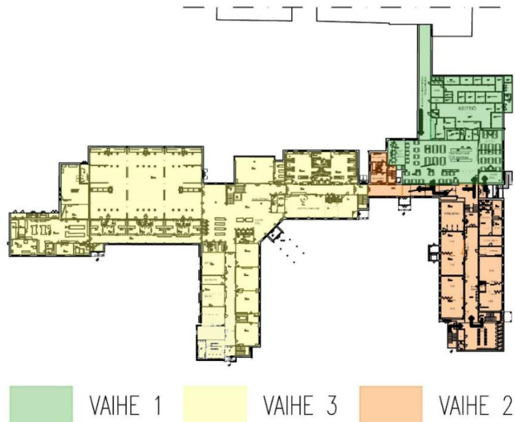
Kuva 5 Rakentamisen vaiheistuskaavio
