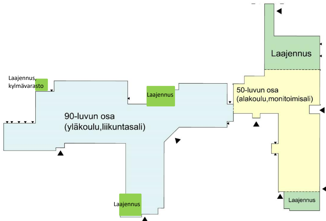
Kuva 3 Koulun rakennusosat
